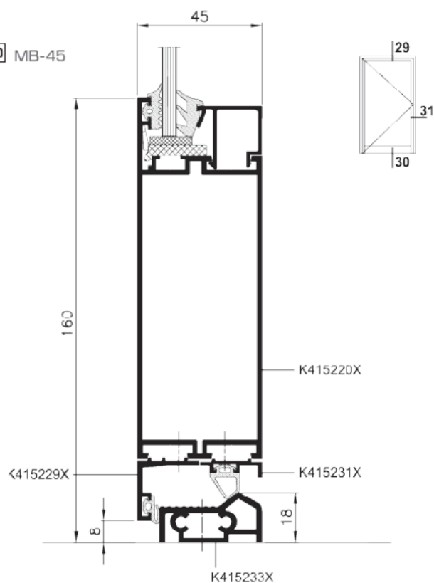
„Standard” szimpla, aktív, kifelé nyíló ajtó - keresztmetszet
