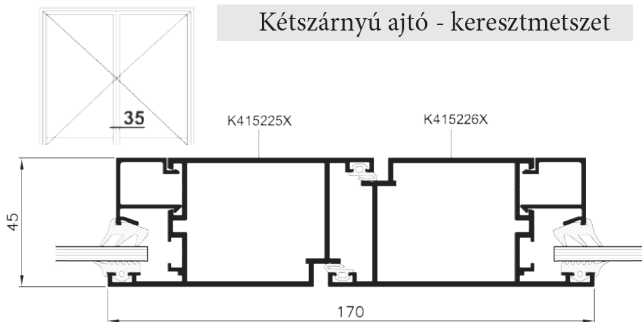
Duplaajtós kirakat - keresztmetszet
