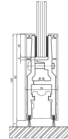
Mobile és ajtószárny – alsó keresztmetszet
