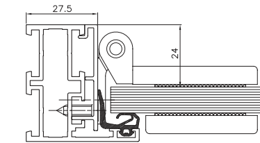
Ajtó – oldalnézet
