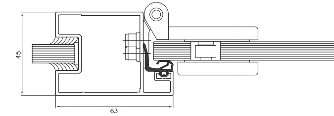
Ajtócsap és felső keresztződ nézete
