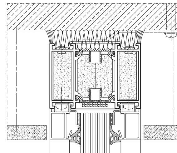
Szilikonnal illesztett üvegfal – felülnézet
