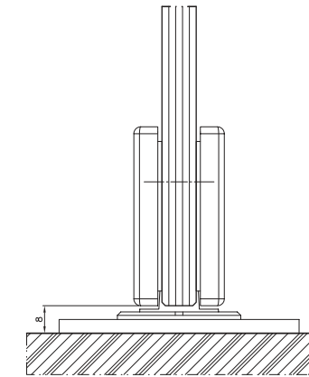
Csupa-üveg ajtószárny – alsó nézet
