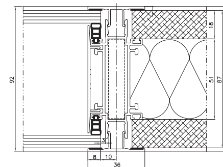
92 mm-es fal – függőleges nézet
