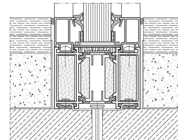
Szilikonnal illesztett üvegfal – alulnézet
