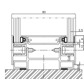
Alsó keresztirúd – nézet
