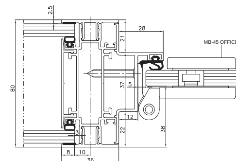
Ajtó – vízszintes nézet
