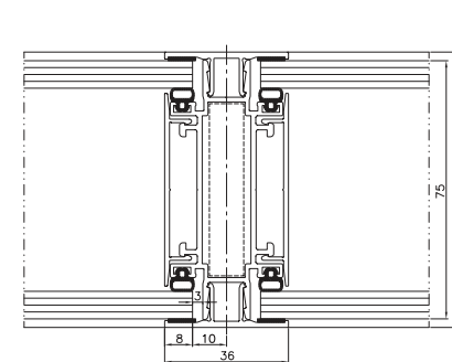
80 mm-es fal – függőleges nézet
